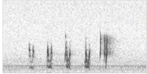
Abb.5 Sonagramm Wachtel 01.06.21
